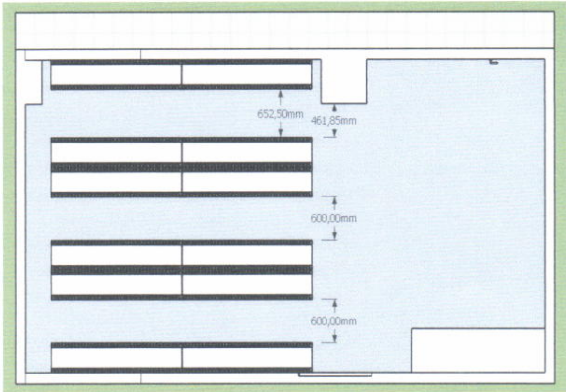
Gambar 3. Tampak atas rak rekam medik
