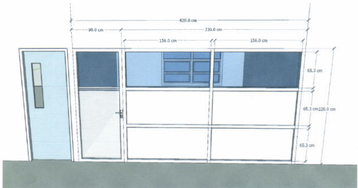
Gambar Rencana dan Ukuran Partisi Perpustakaan 3B
